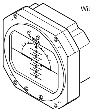
RCA 2610-3-G P/N 102-0403-03-03 P/N 102-0403-05-04
